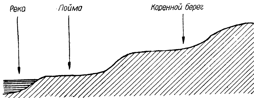
Рис. 4. Разрез речной долины.
