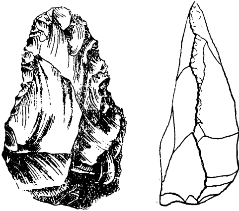
Рис. 6. Ручное рубило.
