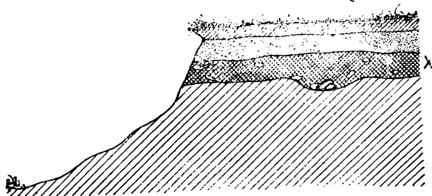
Рис. 1. Разрез почвы с культурным слоем. х — культурный слой.
