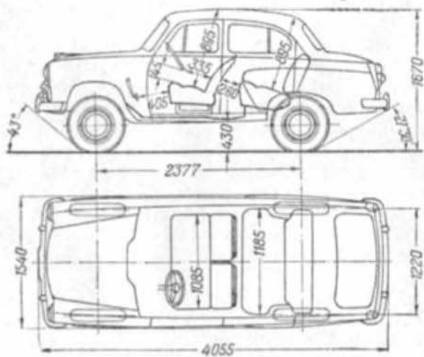
Рис. 2. Габаритные и внутренние размеры автомобиля «Москвич» модели 410
