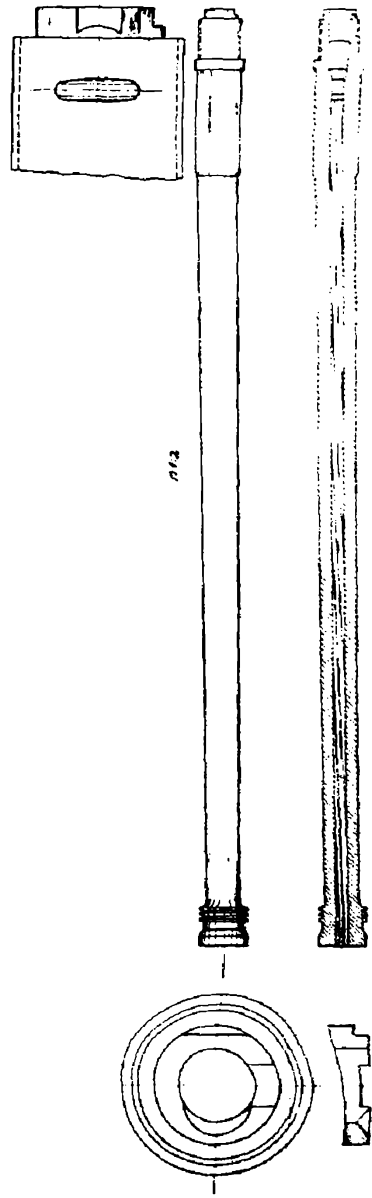
АВИАЦИОННЫЙ ПУЛ. МАДСЕНА
