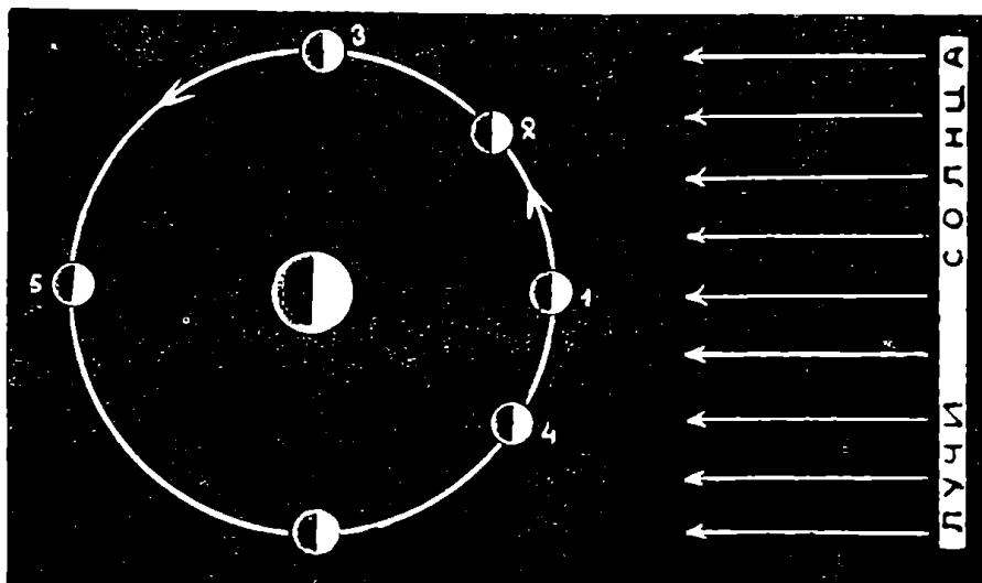
Рис. 1. Фазы Луны.
